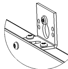
Fästvinkel (närbild)
