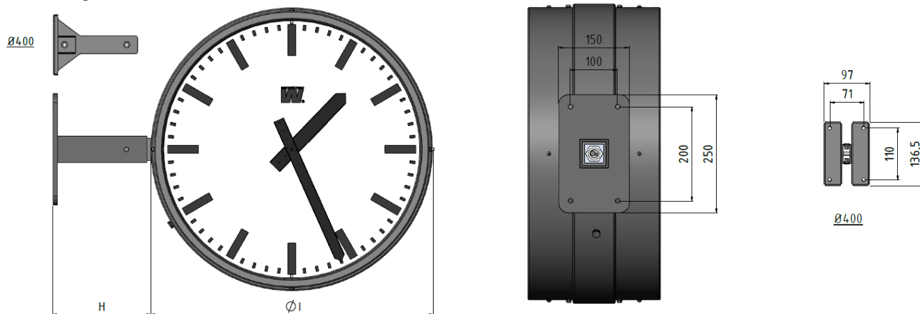
Dubbelsidig Ø 400-900
